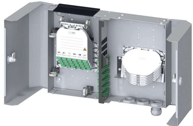
CCM Open Access Gehäuse (Abbildung ähnlich)
