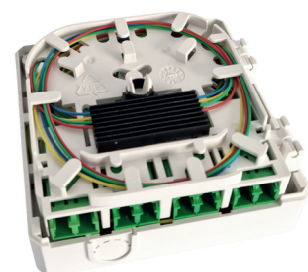
CCM ARCA FTTH XS Anschlussdose bestückt mit 4 LCAPC Duplex Kupplungen
