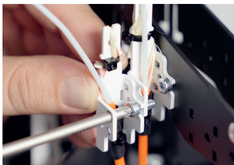
Grafik: Faserführung in der Spleisskassette
