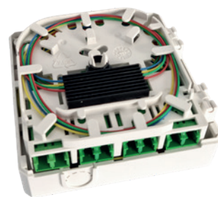
CCM ARCA FTTH Anschlussdose bestückt mit 4 LCAPC Duplex Kupplungen
